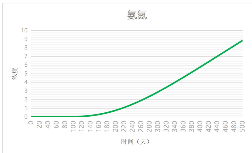
图 6.4-3 跟踪监测井氨氮水质污染物浓度穿透曲线
