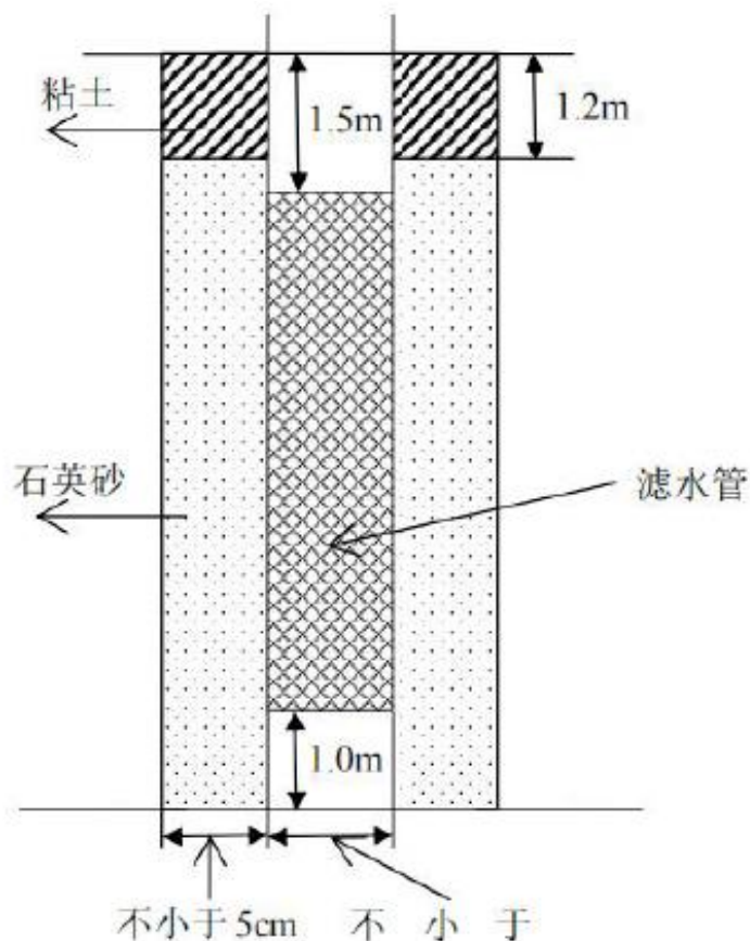
图 6.4-6 地下水监测井结构示意图
