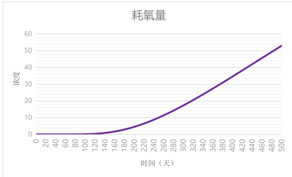
图 6.4-4 跟踪监测井耗氧量水质污染物浓度穿透曲线
