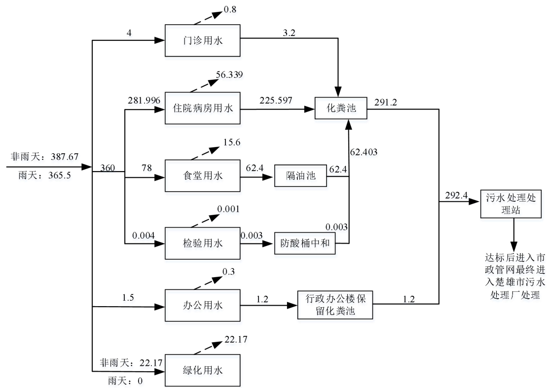
图 4.2-3 项目水量平衡图（m³/d）
