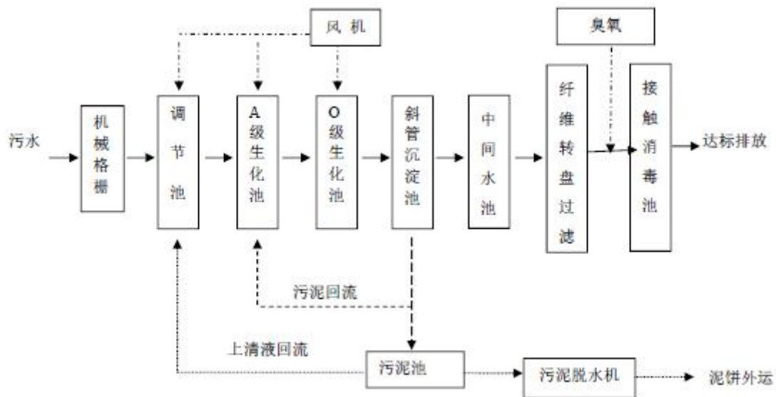
图 7.2-1 项目污水处理站拟采用工艺
