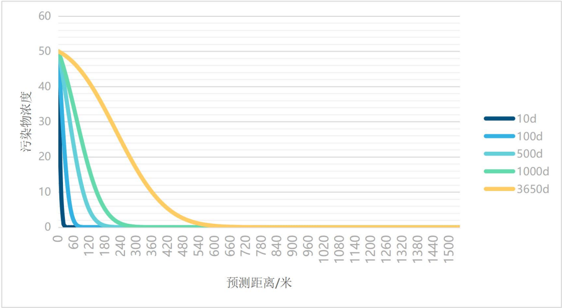
图 6.4-2 项目区下游地下水中耗氧量浓度变化曲线图
