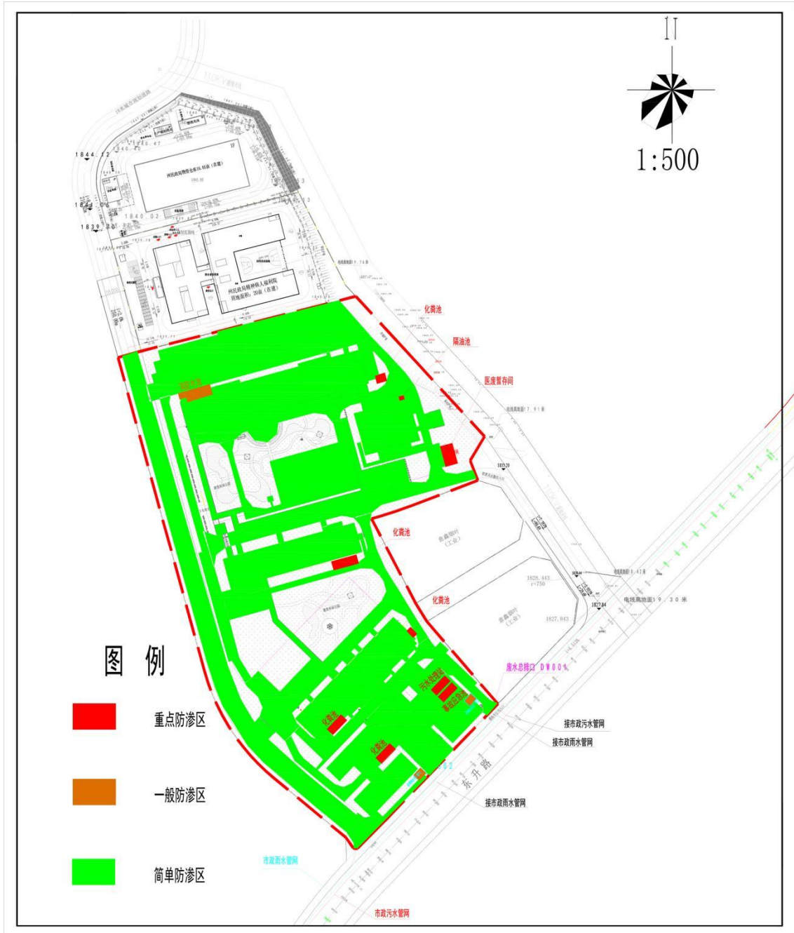
图 6.4-5 项目场地防渗分区图
